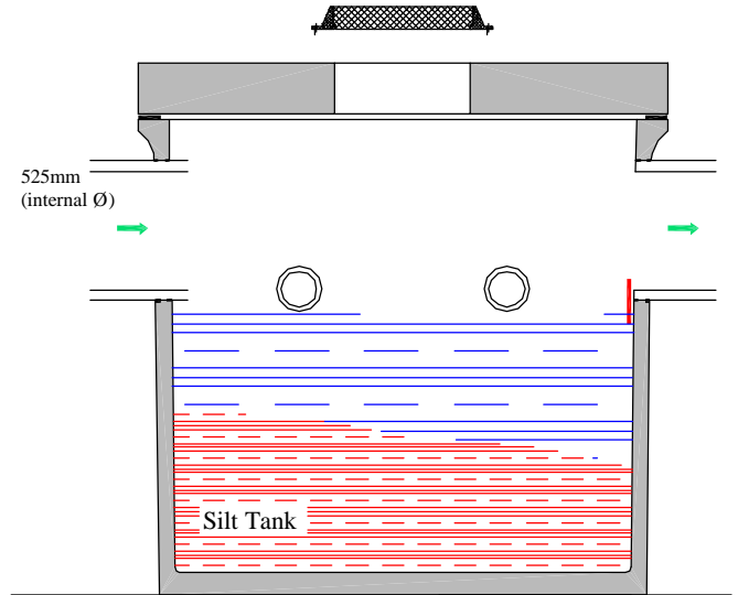
Sec A-A
