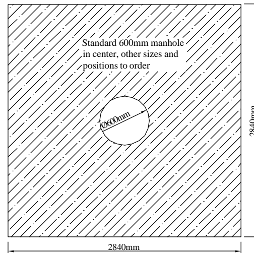
Lid Top Plan
